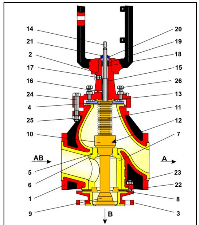
Bild 2 - Schnitt durch ein 3-Wege Ventil BR 1d, ab DN 80 und 3" , Stückliste siehe Tabelle 1 auf Seite 3
