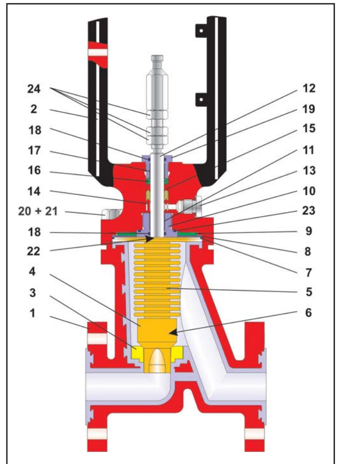
Bild 2 - Schnitt durch ein Stellventil BR 1b => Stückliste siehe Tabelle 1 auf Seite 3
