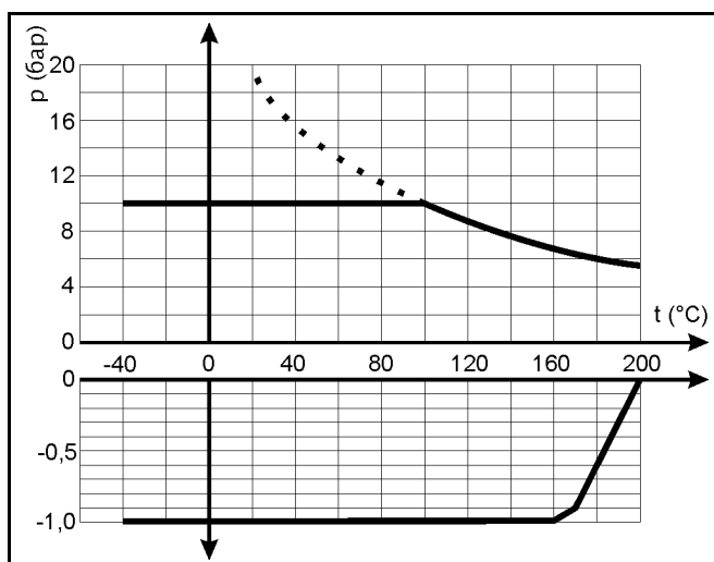
Рис. 4 Диаграмма «Давление-температура»
