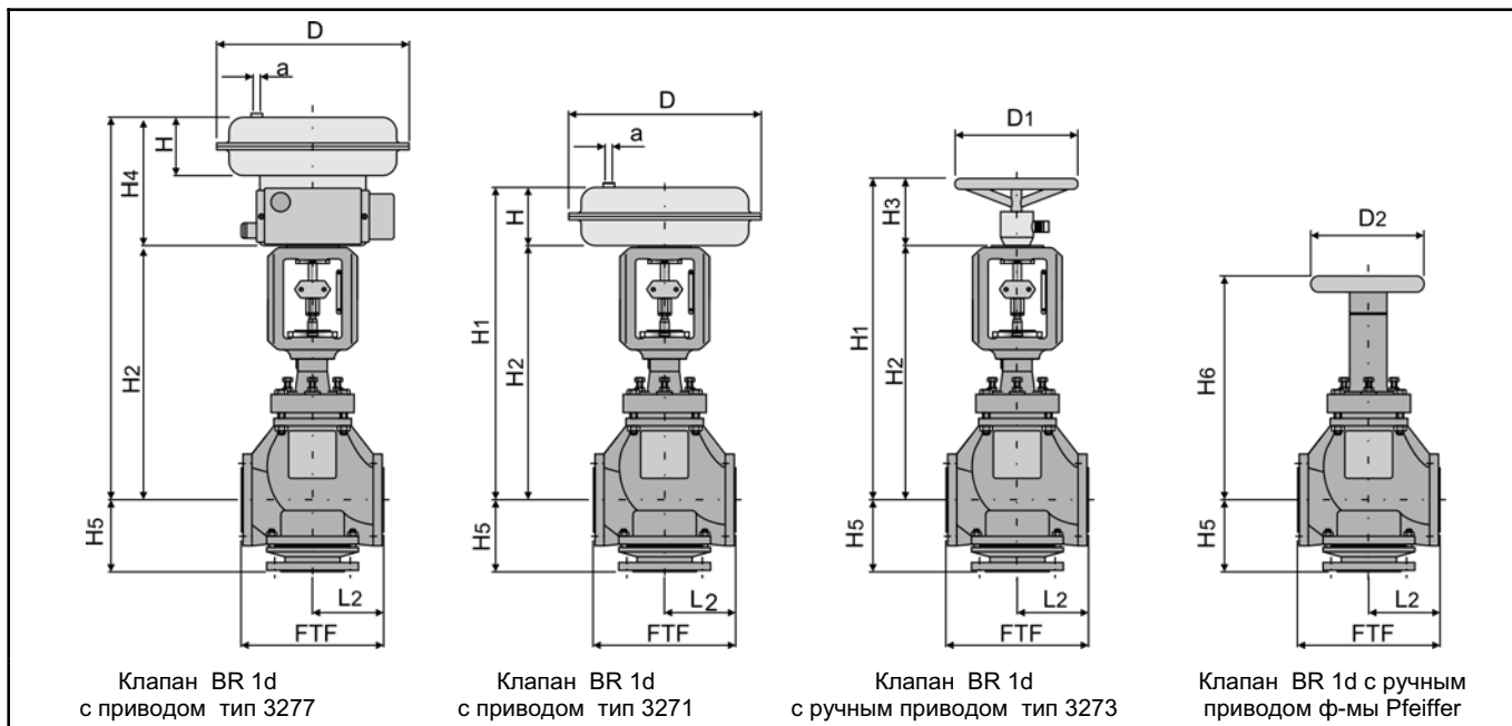
Рис.4 • Размеры
