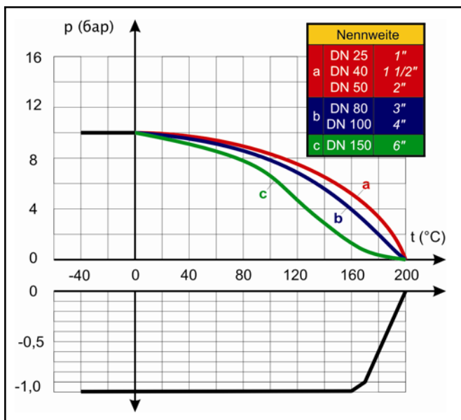
Рис.2 • Диаграмма давление-температура
