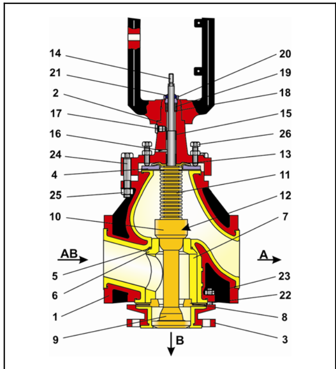
Рис.3 • 3-ходовой распределительный клапан BR 1d
