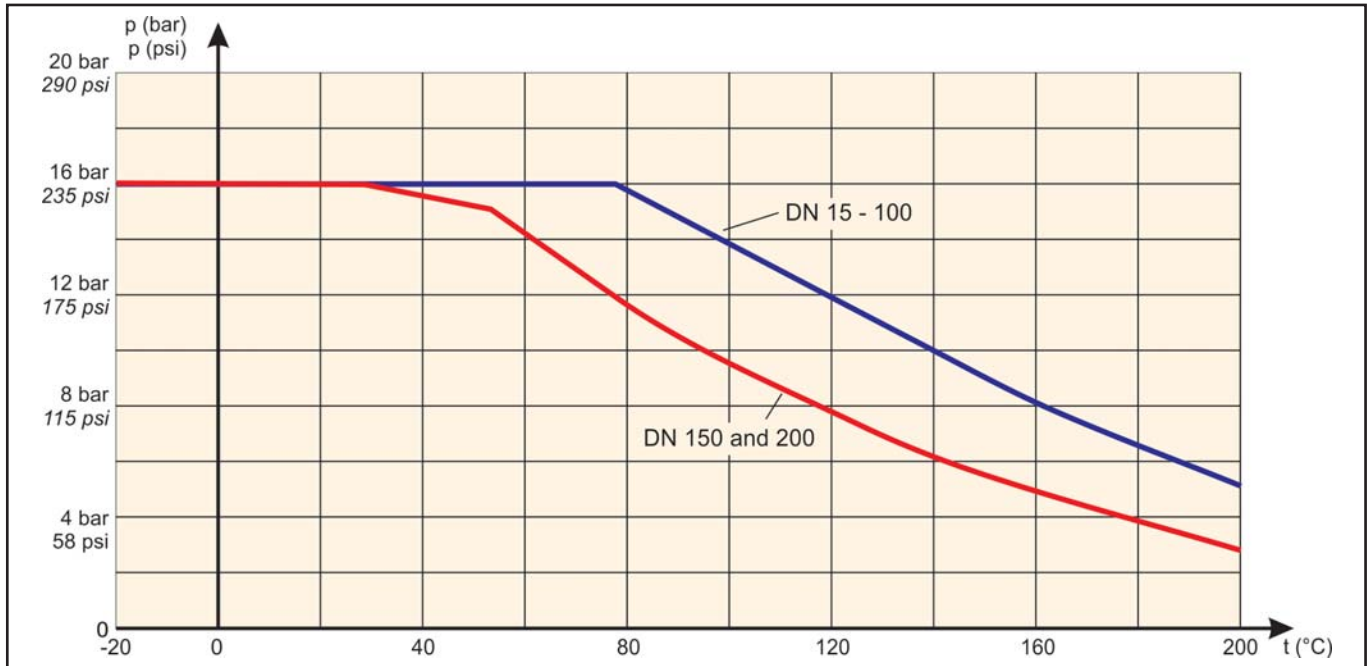
Fig. 6 - Pressure-temperature diagram, PN 16
